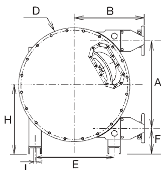
Construction A (flasquée)
